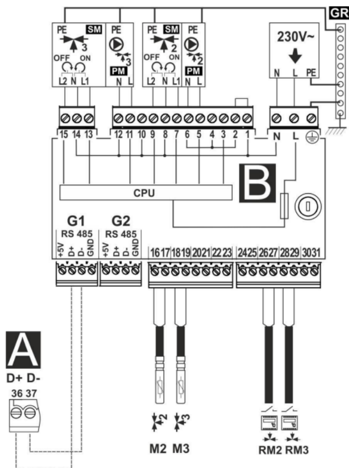
27.2 Elektrické schéma modulu B a C
